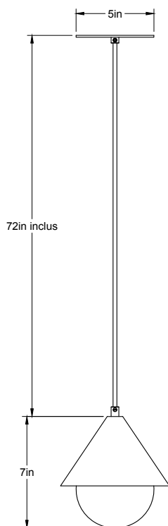
Avant/Front
